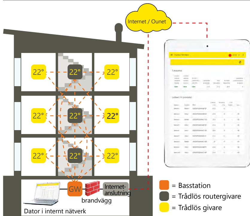
BILD 1 Struktur för trådlöst givarnätverk
